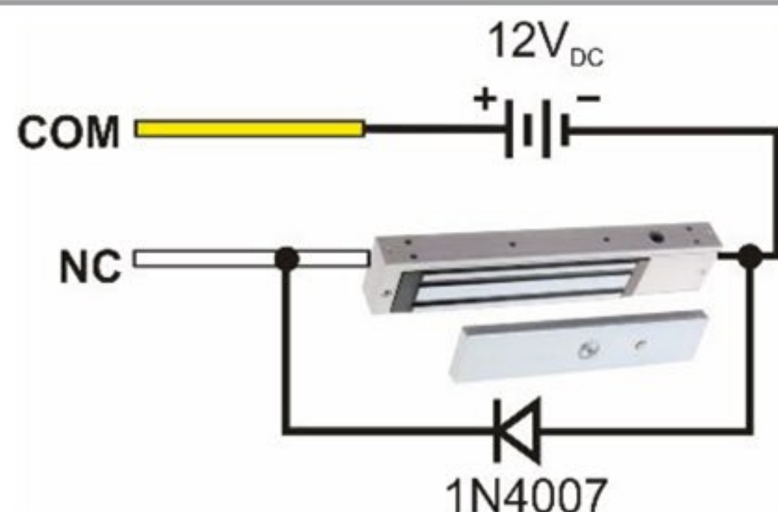
نحوه اتصال کلید به قفل الکترومغناطیسی
