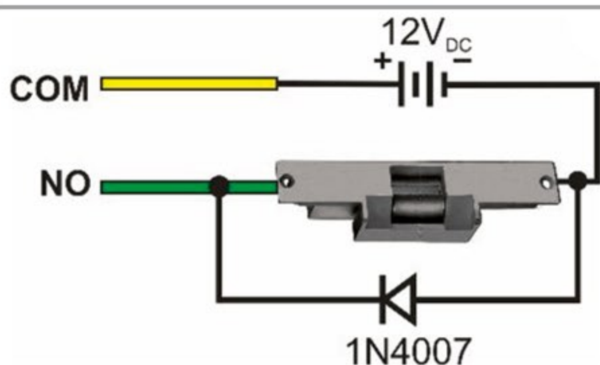
نحوه اتصال کلید به قفل الکتریکی
